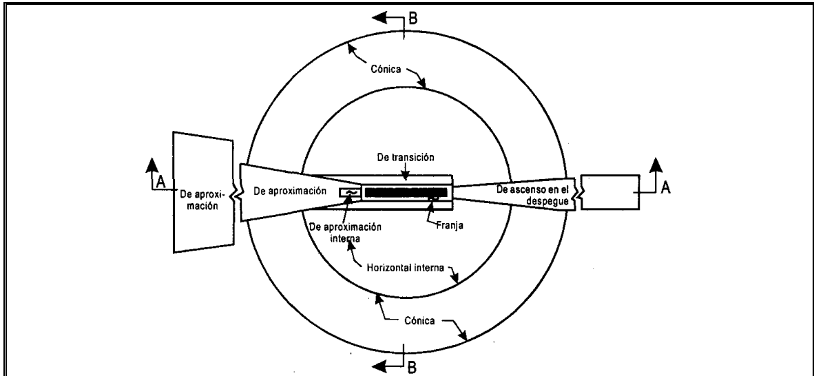
Figura 4 - 1. Superficies limitadoras de obstáculos
