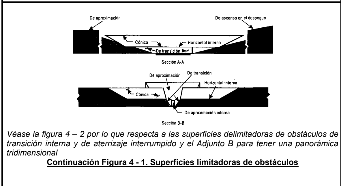
Figura 4 - 1. Superficies limitadoras de obstáculos
